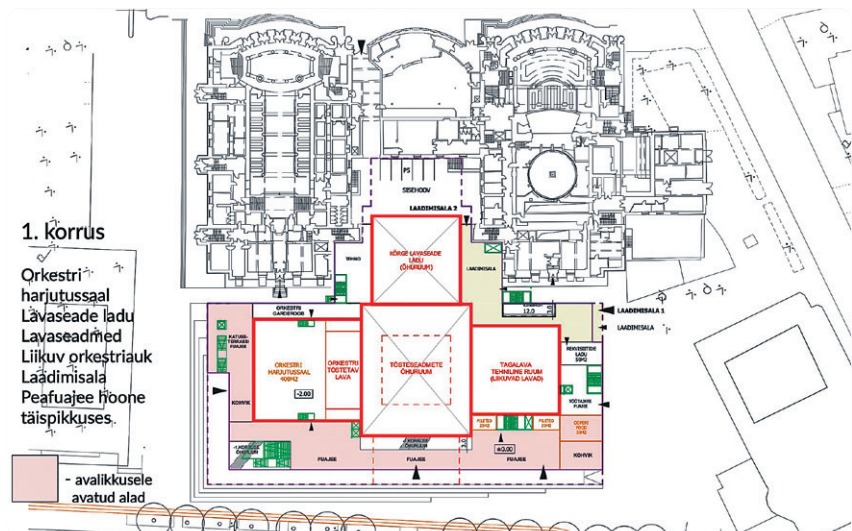
Rahvusoperi juurdeehitise skeem.
